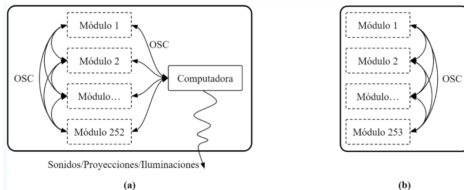
Figura 3. Esquemas de modos de interacción entre los módulos. (a) Modo dirigido, y (b) Modo colectivo.
