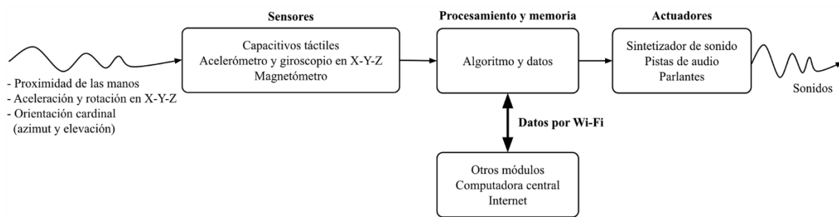
Figura 1. Esquema de un dispositivo sonoro interactivo y modular.
