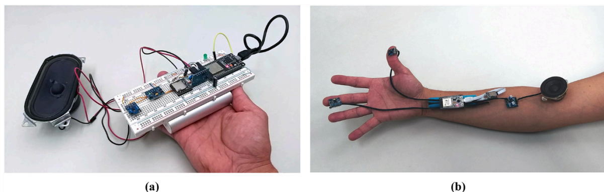
Figura 2. Dos prototipos de módulos sonoros (Fotografías Germán Ito).
